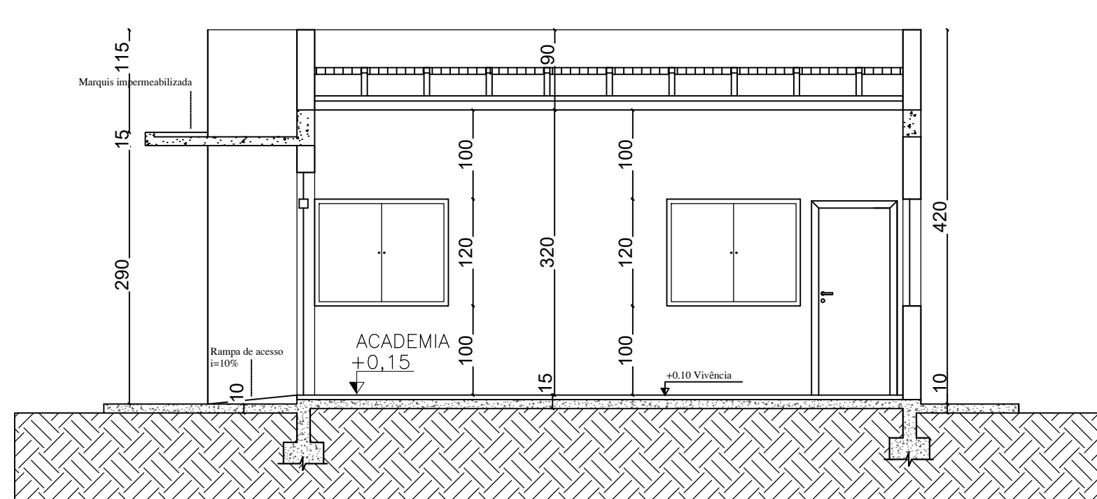
CORTE B-B (ACADEMIA) ESCALA 1:100
