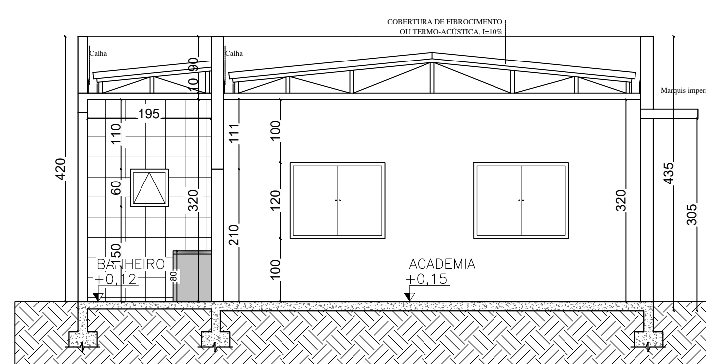
CORTE A-A (ACADEMIA) ESCALA 1:100
